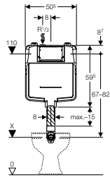
Geberit Sigma concealed cistern 8 cm, 6 / 3 litres
